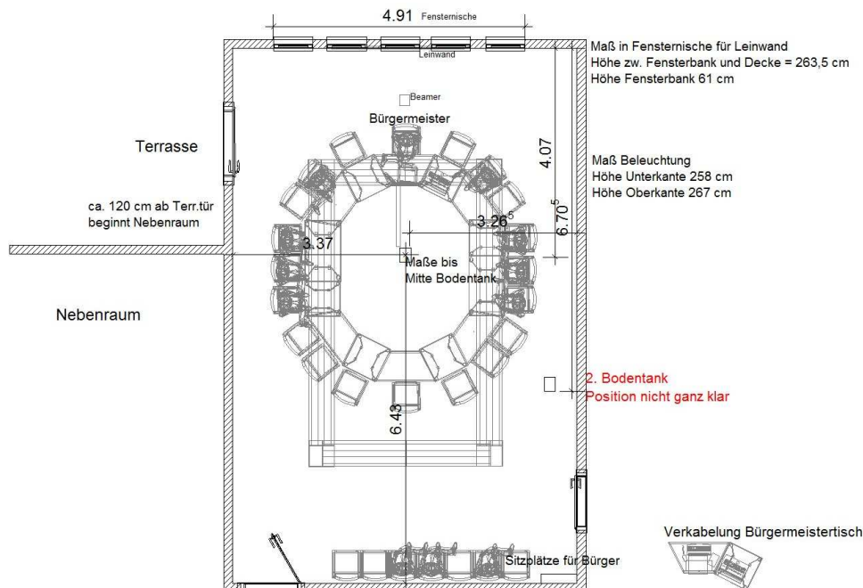
Verkabelungsplanung als Grundrißzeichnung
